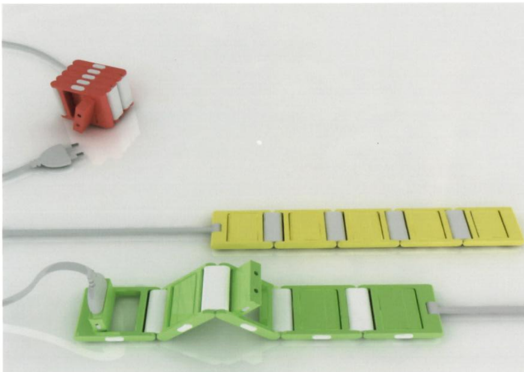
유니버설 멀티탭 Universal Multi-Tap 서준호 Seo, Jun-Ho
