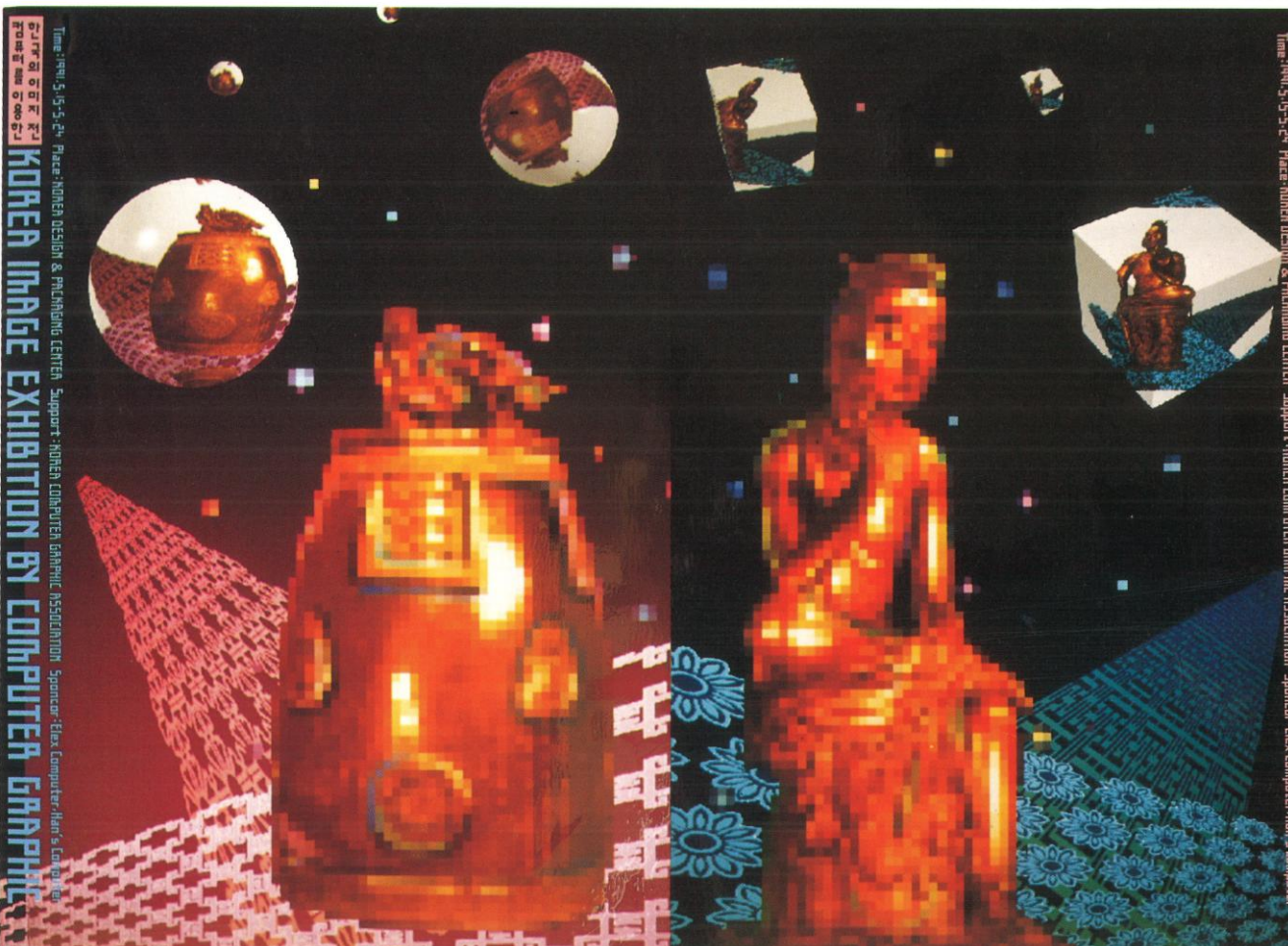
MUN-JA-BO 분자도
