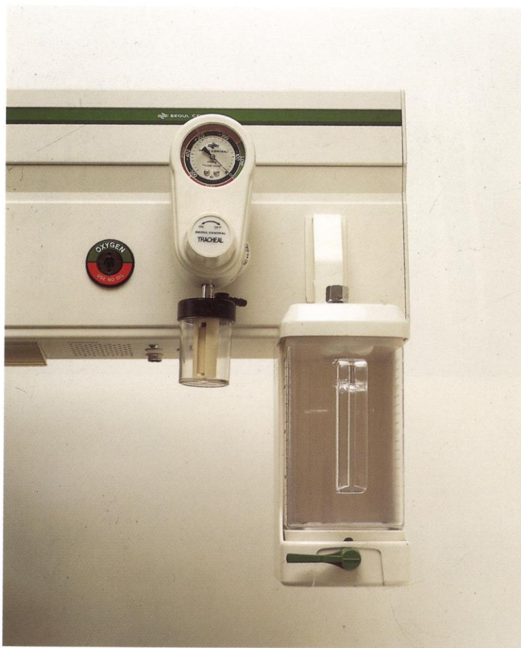
1 의료기 유닛 ICU. BED HEAD UNIT
