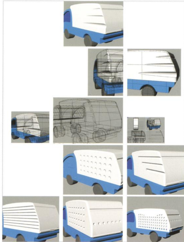
소형 트럭 FRP 적재함 디자인 FRP Housing Concept of Cargo Truck 신명철 Shin, Myung-Chul
