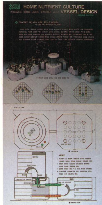
Hydroponic Planter PARK, JUNG-YUN · KIM, SU-JUNG Selected Works 수경재배기 (정액양분배 수경이식기) 박정운 · 김수정 입선작
