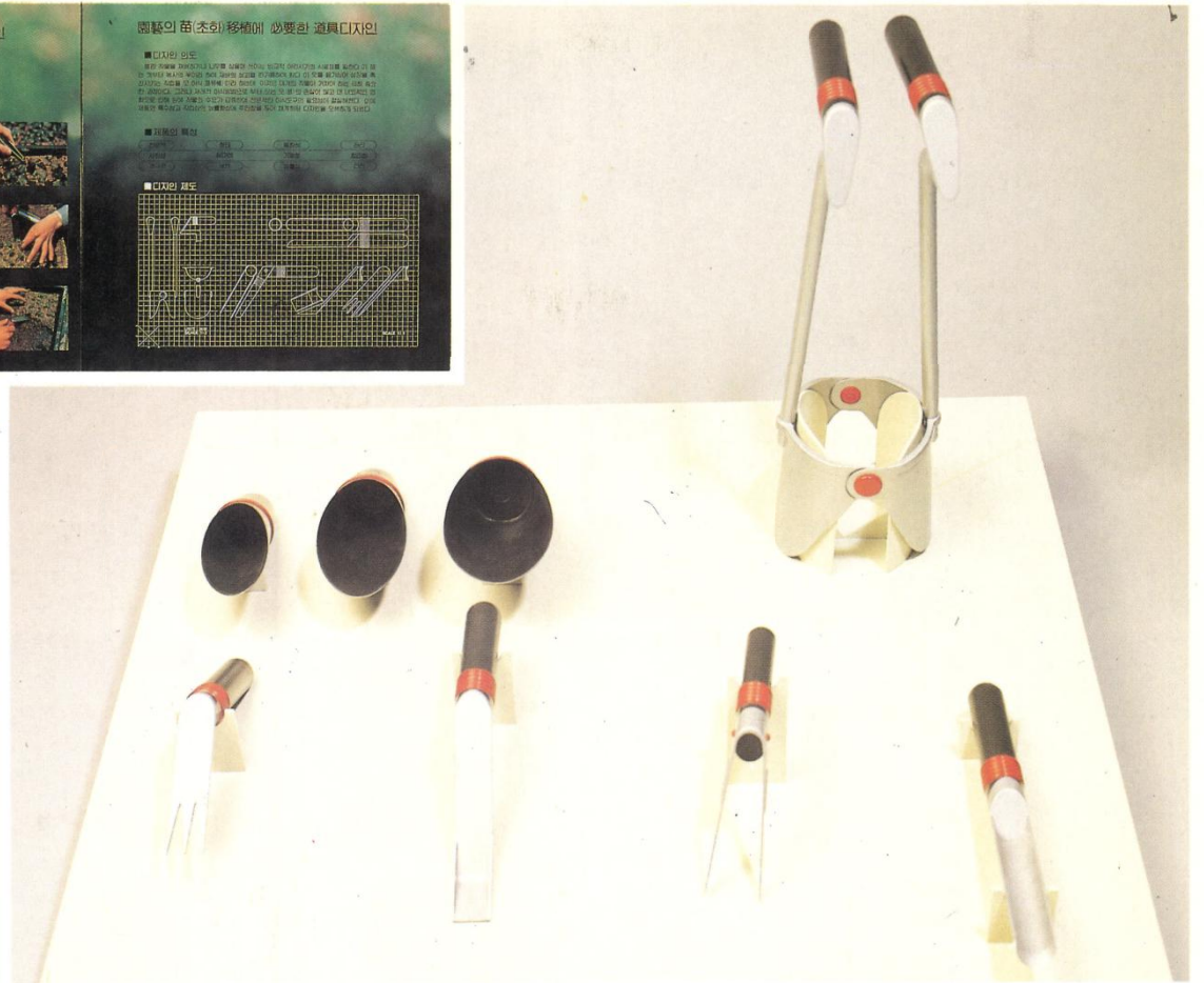
이봉익 김동현 · 이봉익 園藝의 苗(작은)이식용 鋤과 삽의 設計 Selected Works KIM, YONG-HOI · LEE, DONG-SUK Gardening Tools
