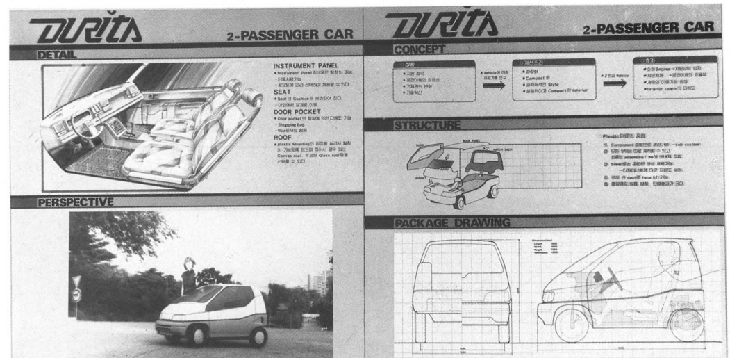
정주현·류인철/2인승 도시형 승용차 디자인 Chung, Joo-hyun. Rhu, In-chul/ 2-Passenger Car
