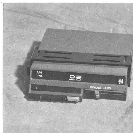
이 재 원 택시 미터기 및 전자 시계
