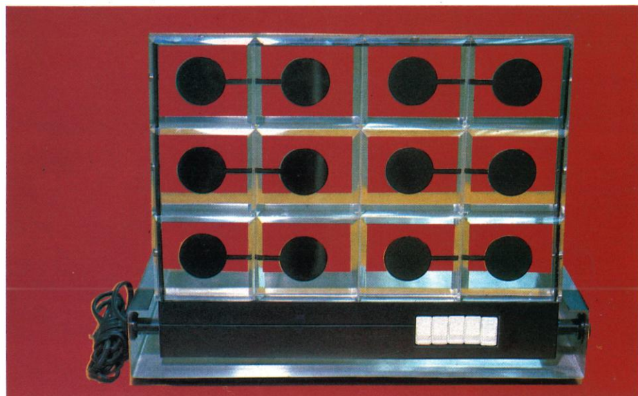
조 종 호 판넬 히이터 디자인 Cho Jong Ho Panel Heater
