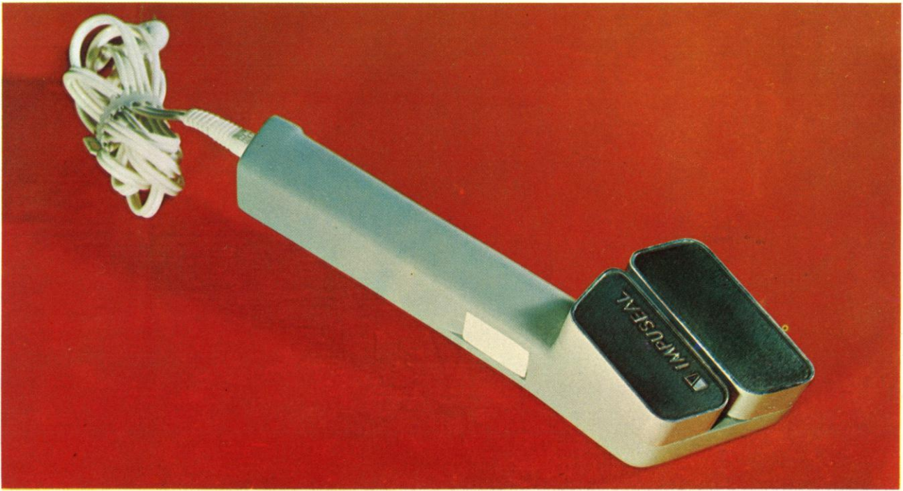
장 호 익 소형비닐접착기 길이 23.5 cm
