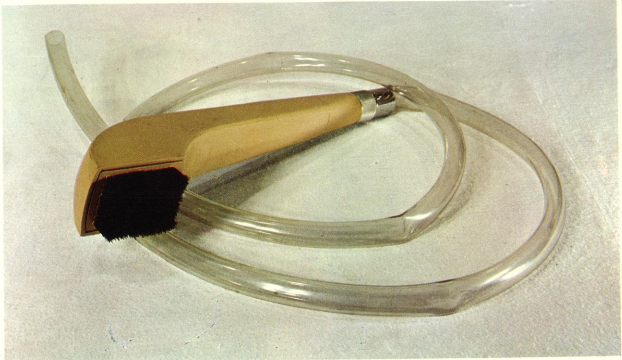
인 인 상 세척용솔 폭 8 cm
