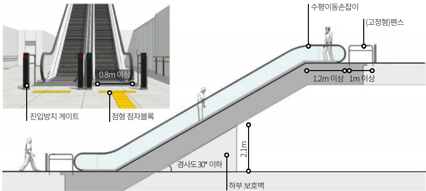
에스컬레이터 설치 예시
