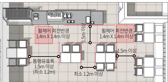
판매공간 통행유효폭 기준
