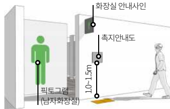
화장실 촉지안내도 설치기준
