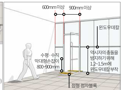
수동문 설치 기준
