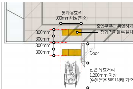
출입구 통과 및 활동공간 유효폭 확보와 점자블록 설치
