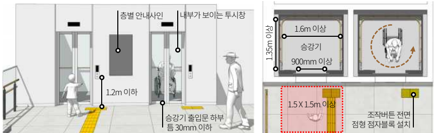
승강기 전면 공간예시 승강기 내·외부 유효공간 설계기준
